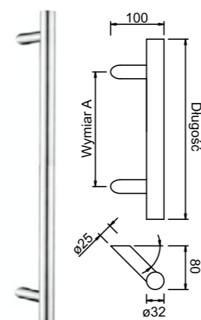
Pochwyt ze stali nierdzewnej 45°
